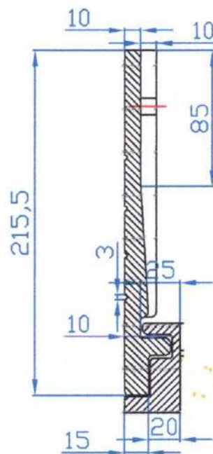
CORTE LONGITUDINAL
